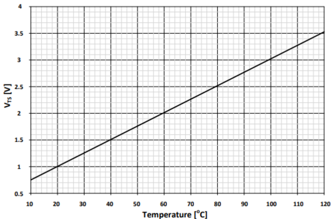
图 6: VOT 输出电压曲线
